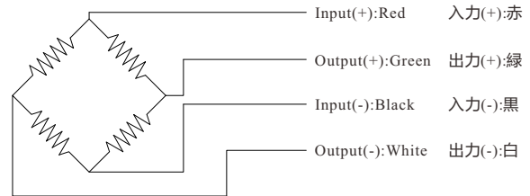
Wiring Diagram/配線図
